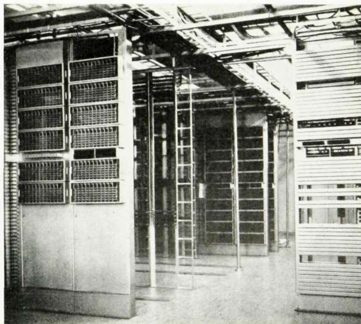
En interiör från den automatiska telefonstationen Sörnäs i Helsingfors, utförd enligt L M Ericssons sidvägssystem med koordinatväljare.
