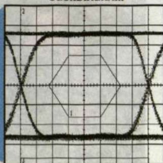
ÖGONDIAGRAM
