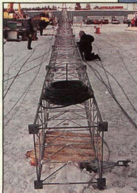
Swesite-masten är monterad och klar att lyfta. Den består av ett antal två meter långa sektioner som skruvats ihop. Varje sektion väger 70 kilo.
