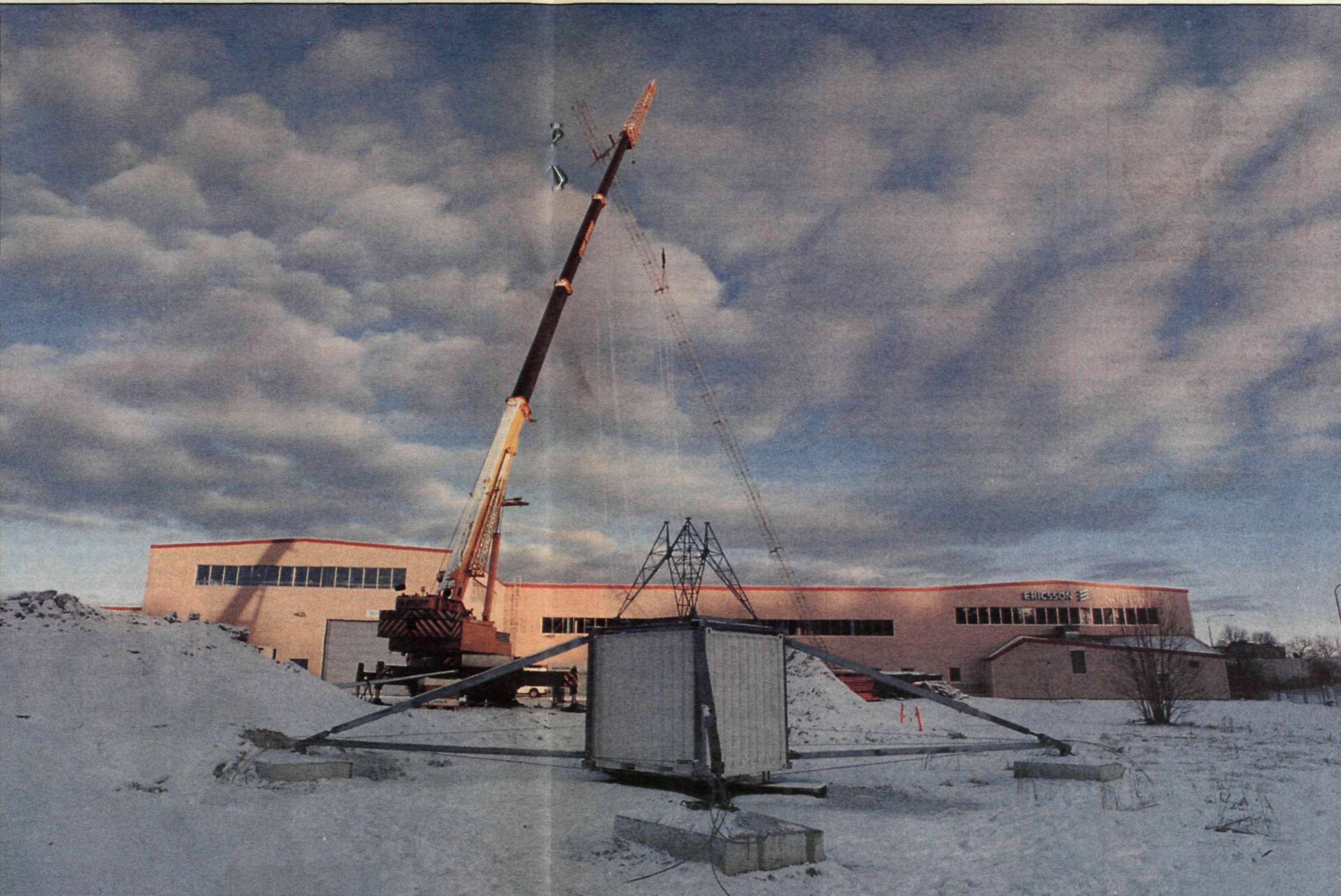
I förgrunden shelter med all erforderlig teknisk utrustning och de två och ett halvt ton tunga fundamenten.
