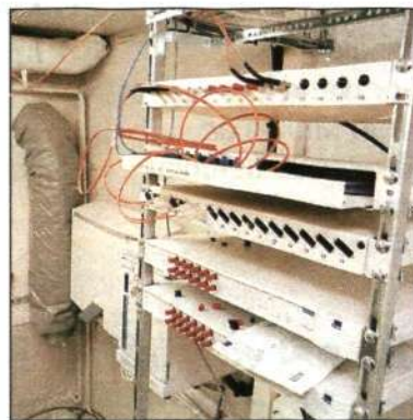
Optisk fiber går till varje lägenhet. Det mesta av tekniken finns i husets källare vilket underlättar underhållet. Detta är verklighet i IT-huset i Vällingby utanför Stockholm.
