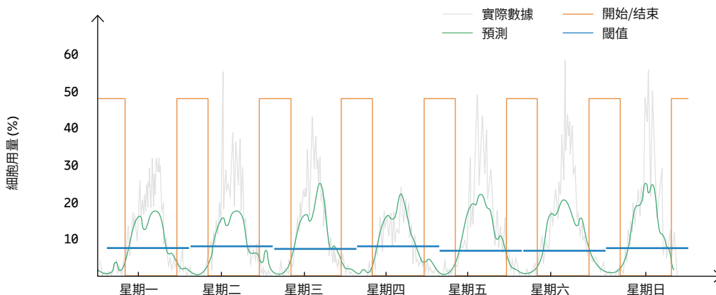
圖7：增強MIMO睡眠模式的人工智慧流量預測
