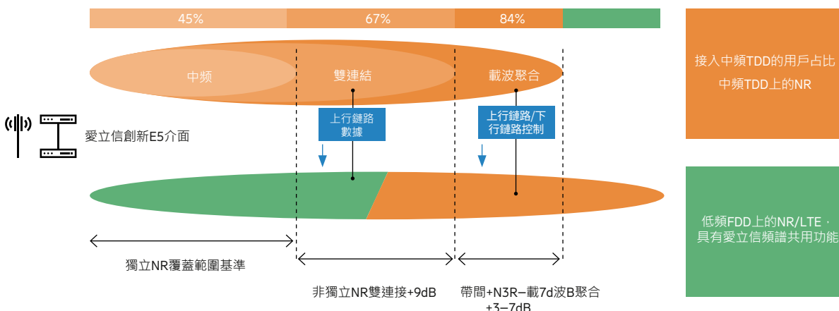
圖8：將5G中頻與低頻的愛立信頻譜共用功能整合在一起
