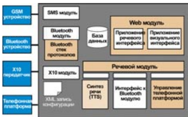
Рис. 18. Архитектура системы
