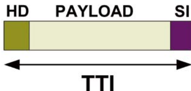
Slika 13. Prikaz E-DPDCH kanala
